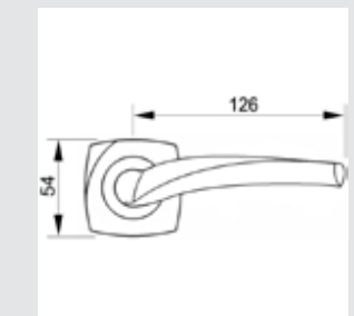
00R6853.000.** Door handle on roses
